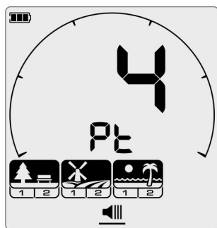
Obrázovka pro nastavení výšky prahu - režimy Park, Field a Beach.
